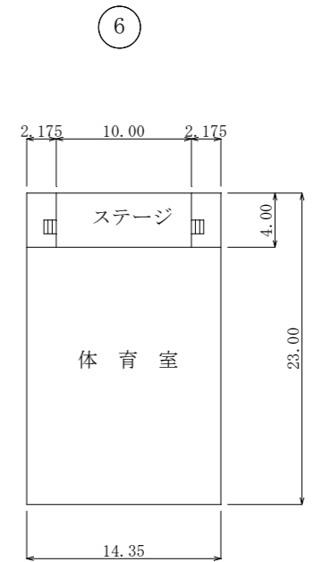
屋内運動場 S
