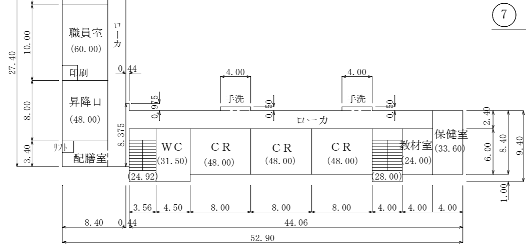
⑦ 2階 平面図 R
