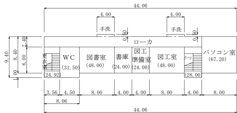
⑦ 1階 平面図 R 教室棟
